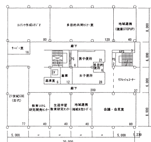
2階平面図 S=1/400
