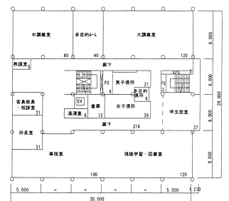
3階平面図 S=1/400
