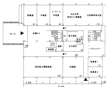
1階平面図 S=1/400
